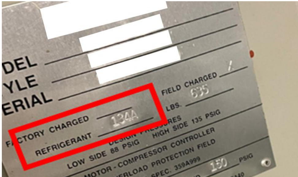
圖 2-8、冰水主機銘牌範例
