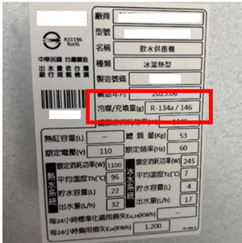
圖 2-9、冰溫熱飲水機銘牌範例
