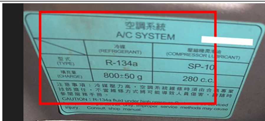
圖 2-10、車用冷媒銘牌範例
