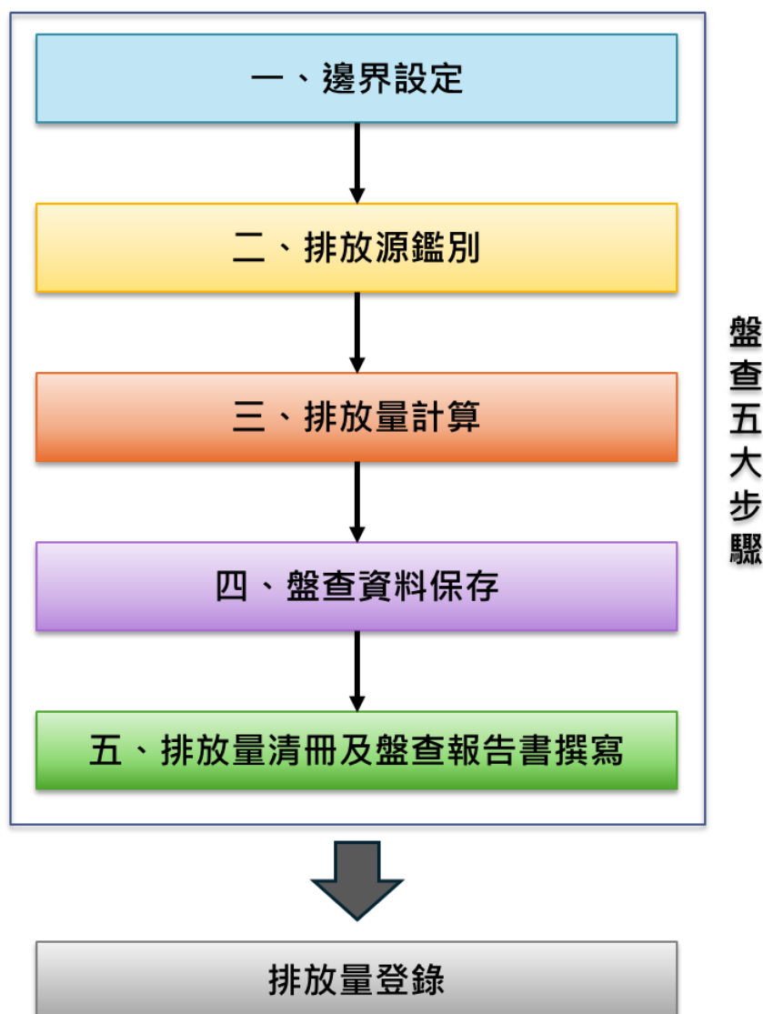
圖 2-1、溫室氣體排放量盤查作業步驟（醫院適用）
